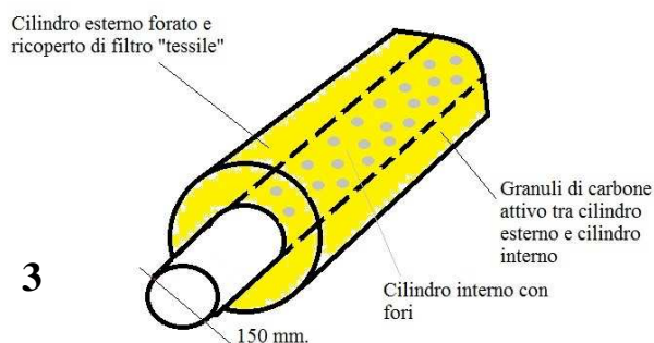
Tra cilindro interno e cilindro ext. granuli di carbone attivo
