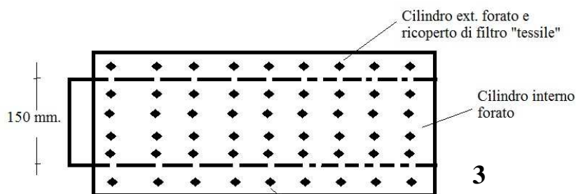
Tra cilindro interno e cilindro ext. granuli di carbone attivo
